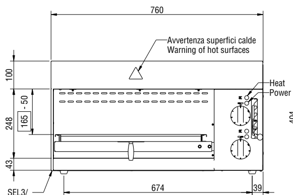
Alzado
